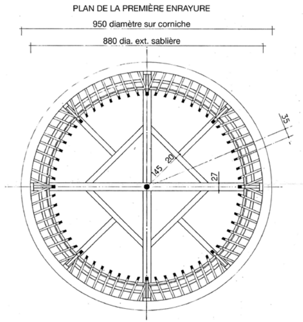
Vue en coupe horizontale de la charpente du donjon central
