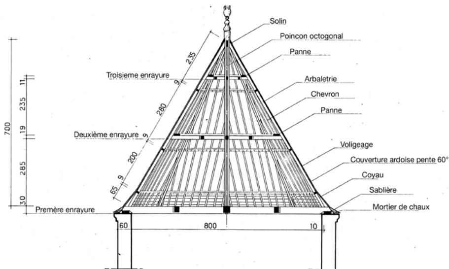
Vue en coupe verticale de la charpente du donjon central
